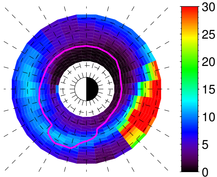
Tz, keV
